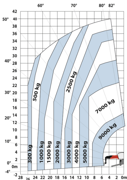
Machine sur stabilisateurs abaissés avec crochet 9000 kg (Métrique)
